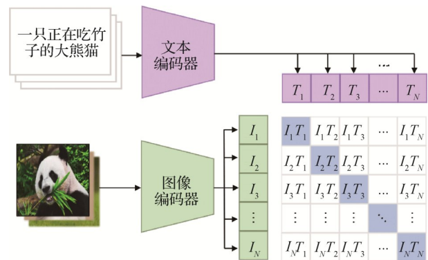
图3 基于对比学习的CLIP模型(Radford等,2021)
