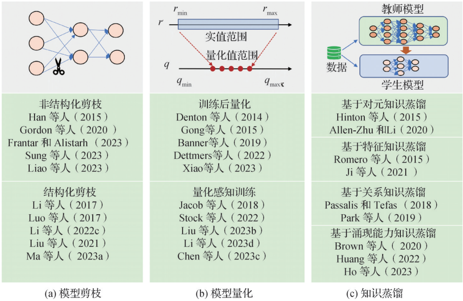
图4 大模型小型化典型方法
