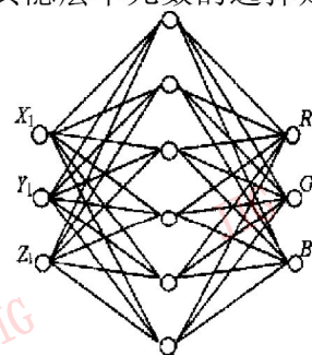
图 5 CRT 的网络结构
