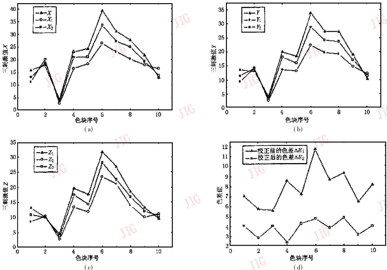
图7 校正前后三刺激值、色差对比曲线
