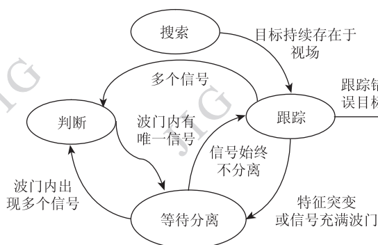
图12 跟踪状态转换关系
