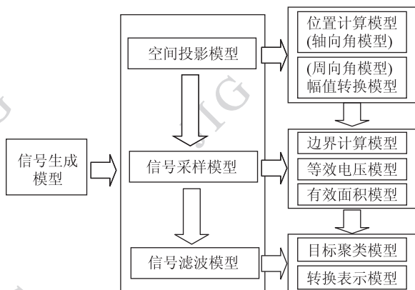
图 6 仿真框图
