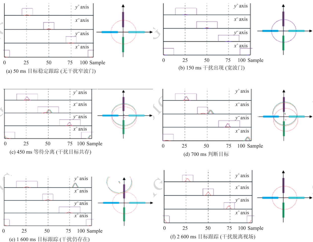
图 16 跟踪过程中探测器效果 Fig. 16 Result of tracking process
