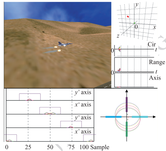
图15 仿真平台 Fig. 15 Simulation platform
