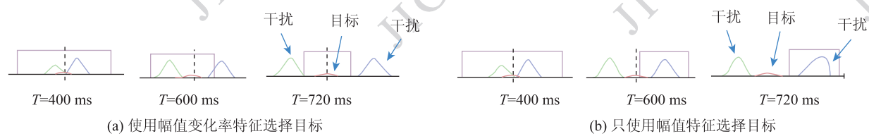
图 17 不同特征的目标选择效果对比 Fig. 17 Comparison of target selection result with different characteristics
