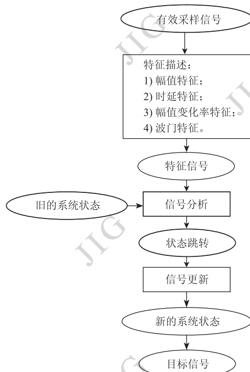
图13 跟踪算法流程
