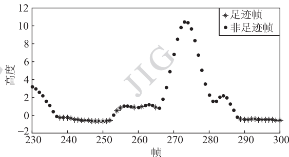
图3 未窗口化样本聚类结果中的足迹标签抖动实例
