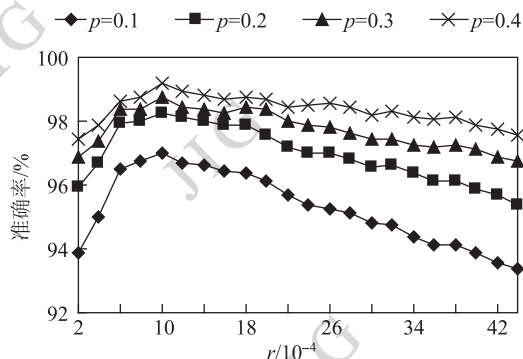
图6 样本方差阈值 r 和模糊时段 p 对整体准确率的影响
