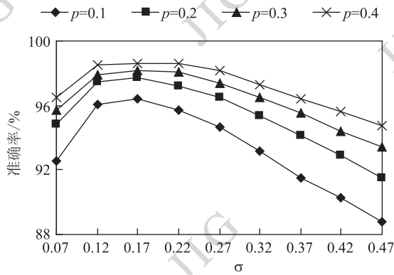
图 8 高斯核函数尺度参数 \sigma 对整体准确率的影响 Fig. 8 Effect of scaling parameter \sigma of Gaussian kernel function on global accuracy rates
