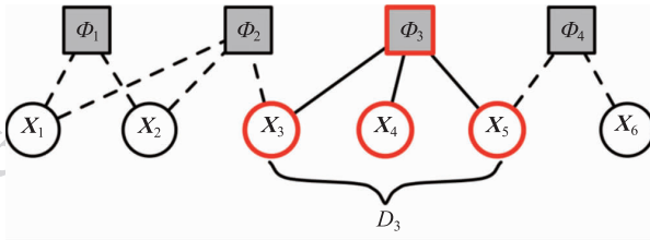
(b) 因子图模型
