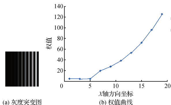
图 1 在不同灰度突变下的权值曲线
