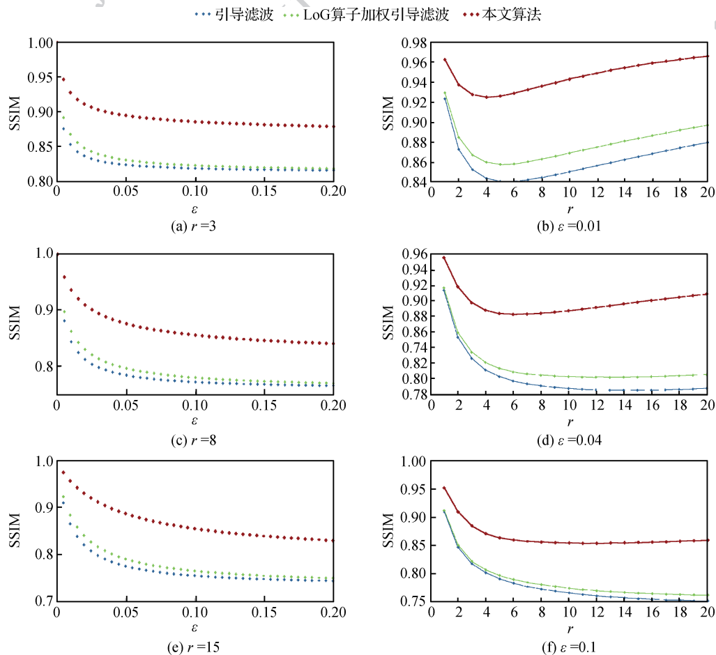
图4 不同滤波方法的图像平滑效果 SSIM 曲线对比
