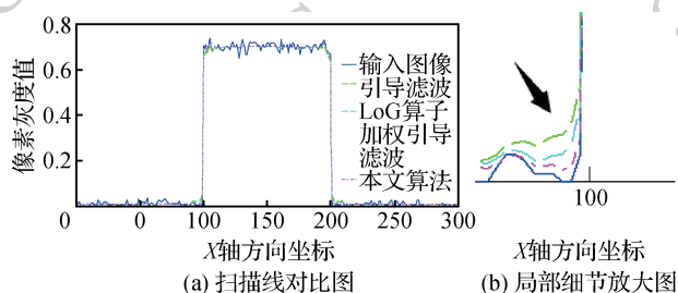
图2 不同滤波方法时输入信号的扫描线对比图
