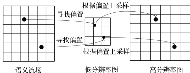
图5 语义流对齐过程
