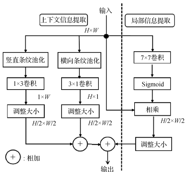
图3 特征聚合下采样模块
