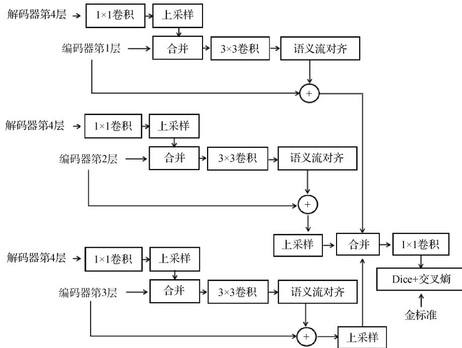
图4 密集语义流监督模块
