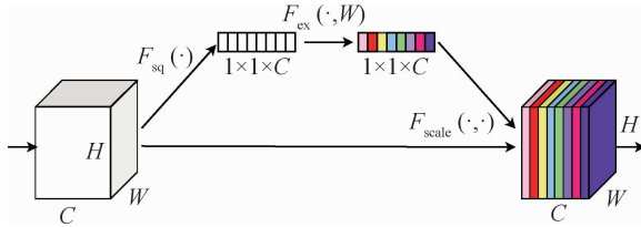
图 2 SE 操作示意图
