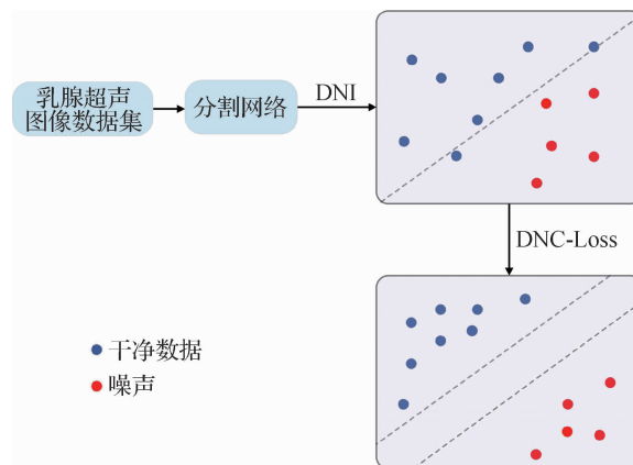
图5 DNC-Loss 对噪声的抑制和对困难样本的挖掘
