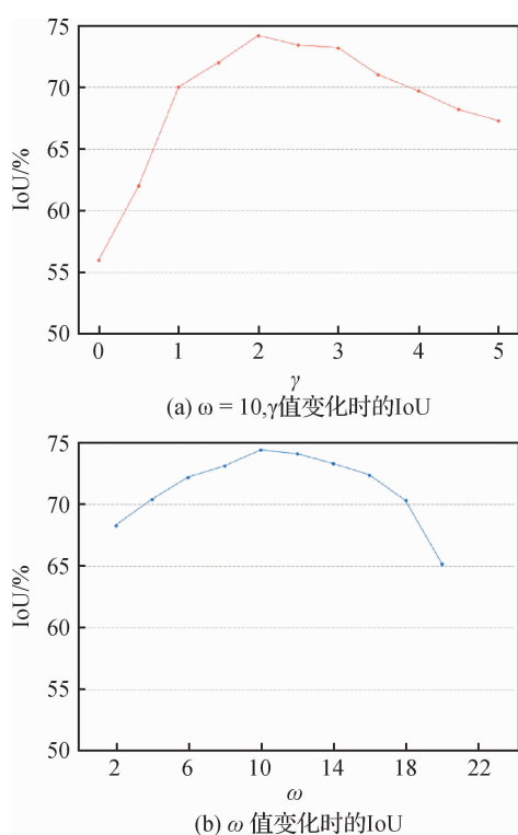
图7 不同的 \omega 和 \gamma 取值在测试集上的IoU
