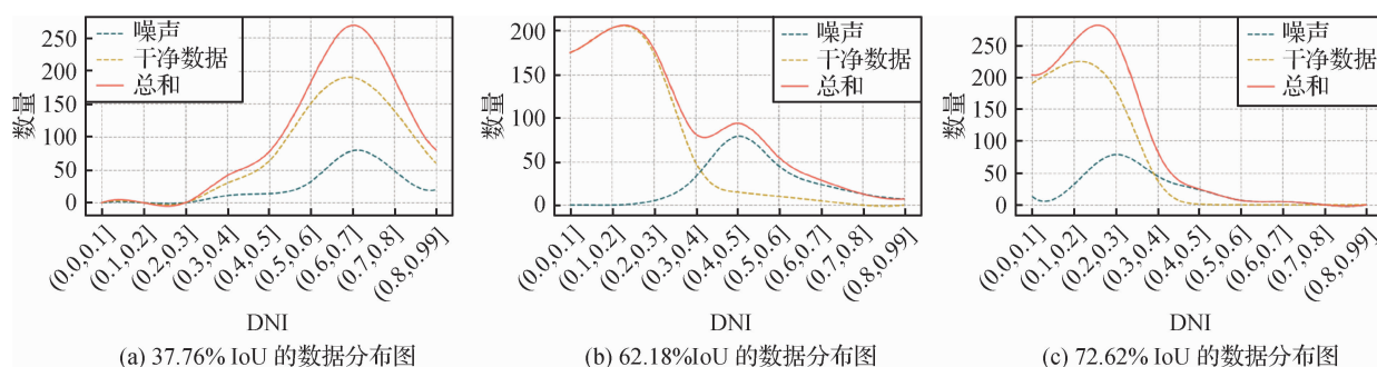
图4 干净样本和噪声在不同训练阶段的DNI分布图
