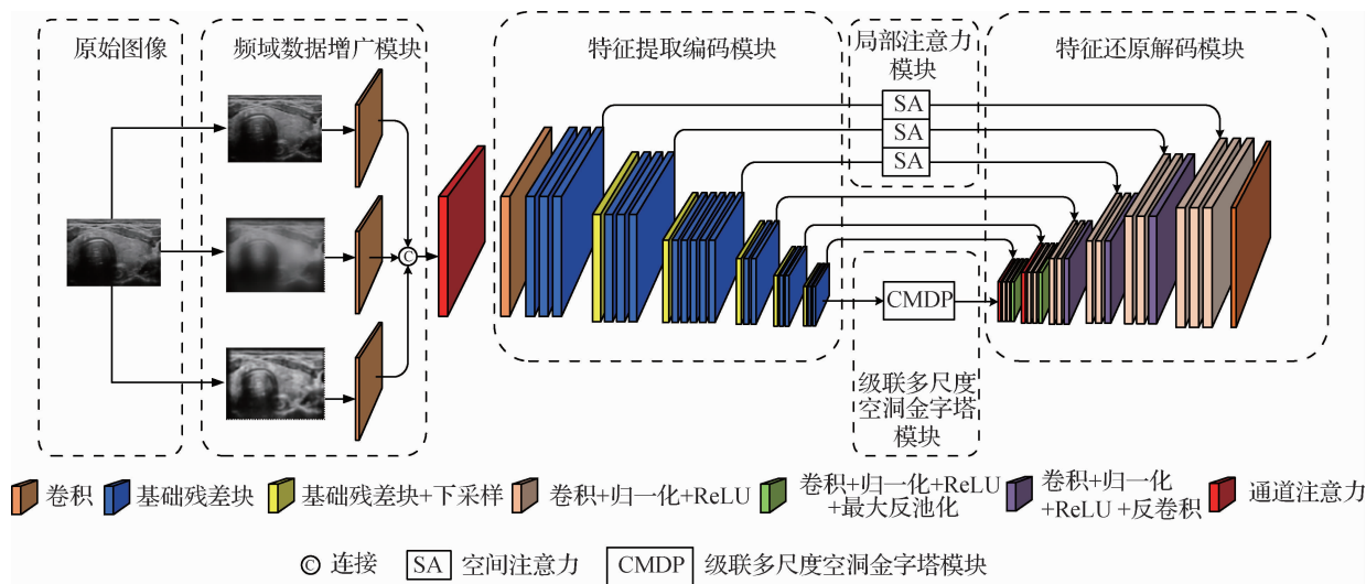
图 1 网络结构图
