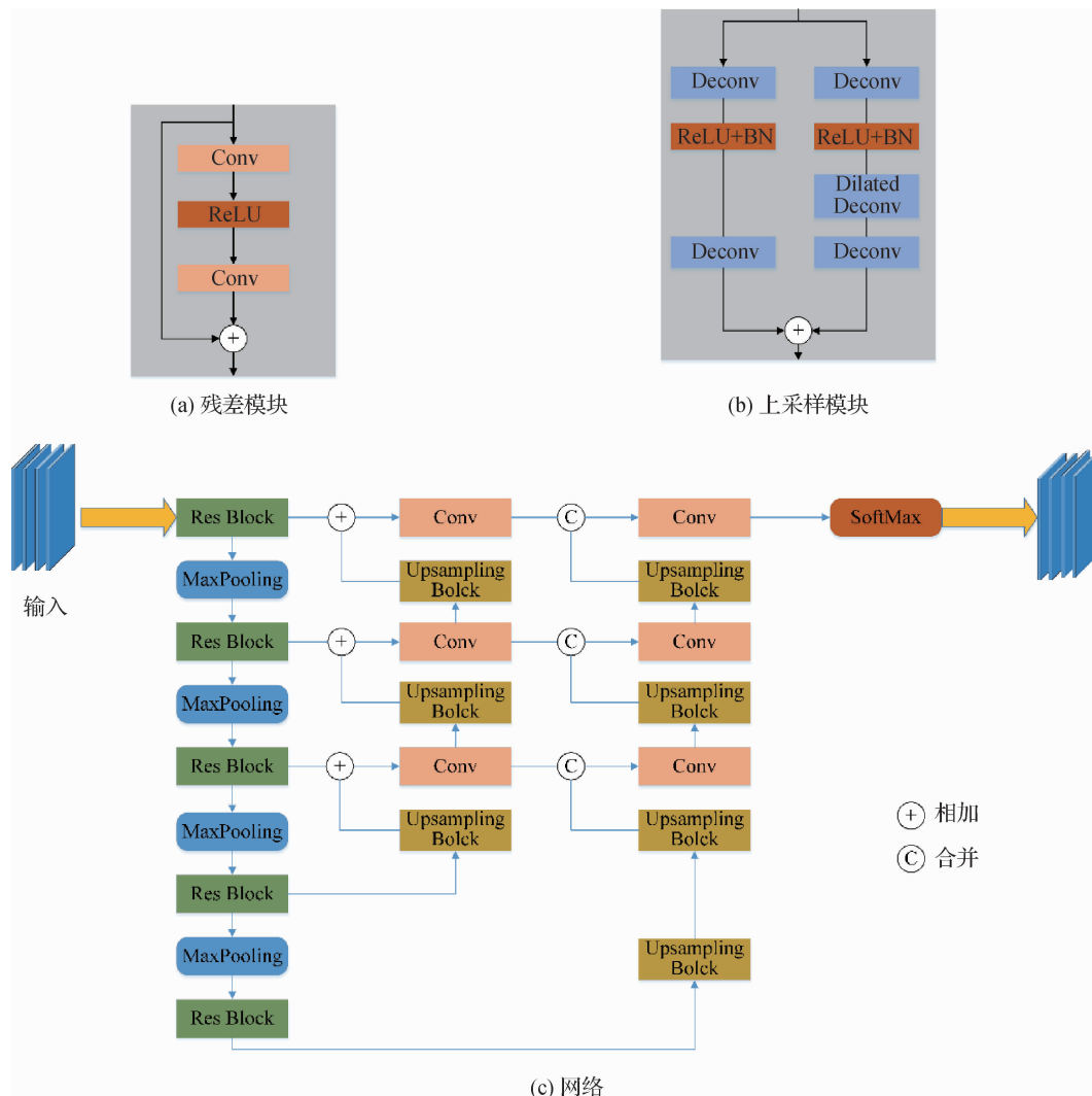
图 2 网络结构
