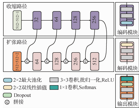
图 4 改进后的 U-Net 结构
