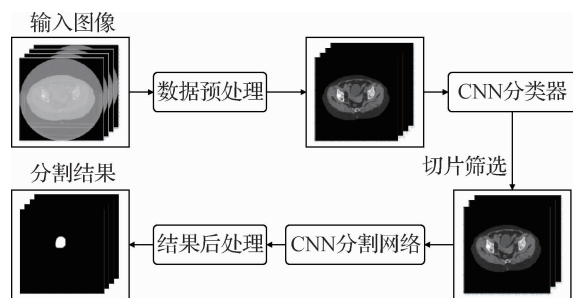
图1 放疗危及器官自动分割框图
