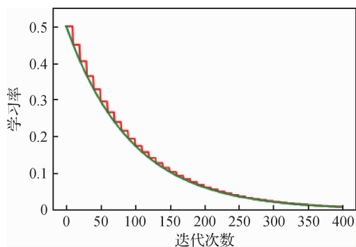
图 3 反时限衰减
