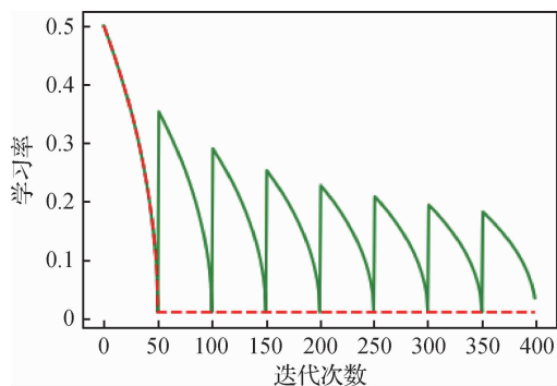
图 2 多项式衰减
