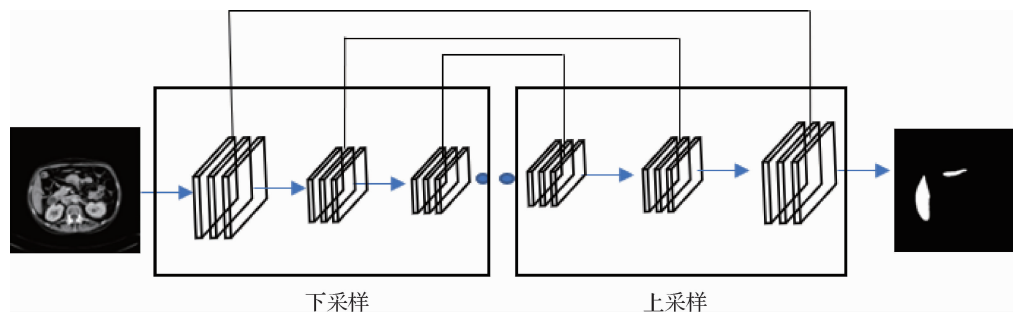
图 5 基于全卷积网络的肝脏肿瘤 CT 图像分割方法基本架构
