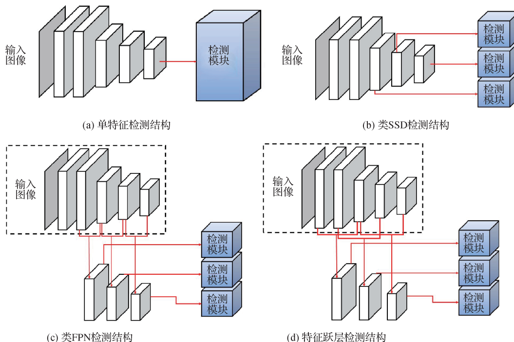
图 3 特征融合检测发展结构图
