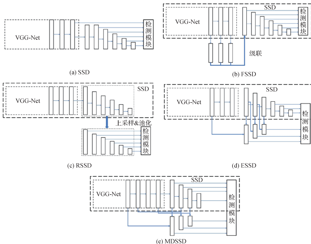
图4 SSD 系列结构特征融合模式示意图
