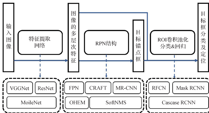
图2 RCNN 的基本结构及改进结构图
