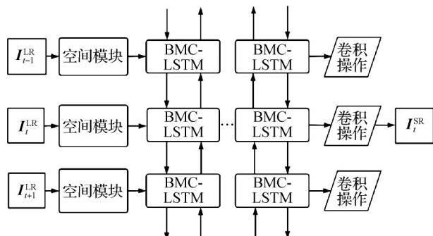
图 28 STCN 的网络结构 (Guo 和 Chao, 2017)
