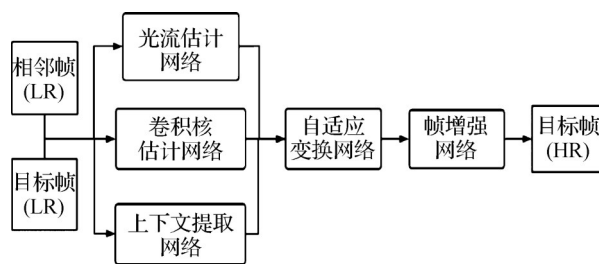
图 18 MEMC-Net 的网络结构(Bao 等,2019b)
