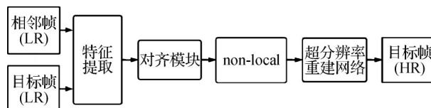
图22 DNLN的网络结构(Wang等,2019a)
