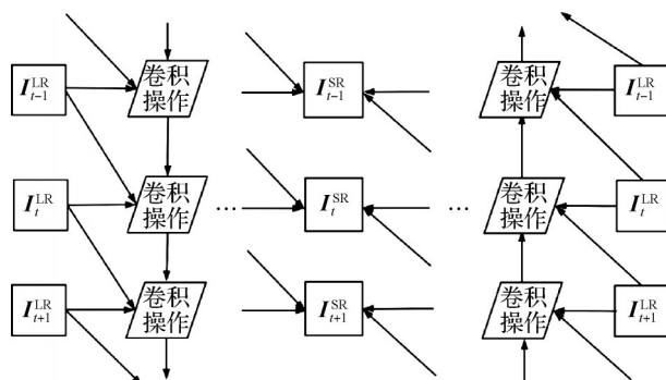
图 29 BRCN 的网络结构 (Huang 等, 2018)
