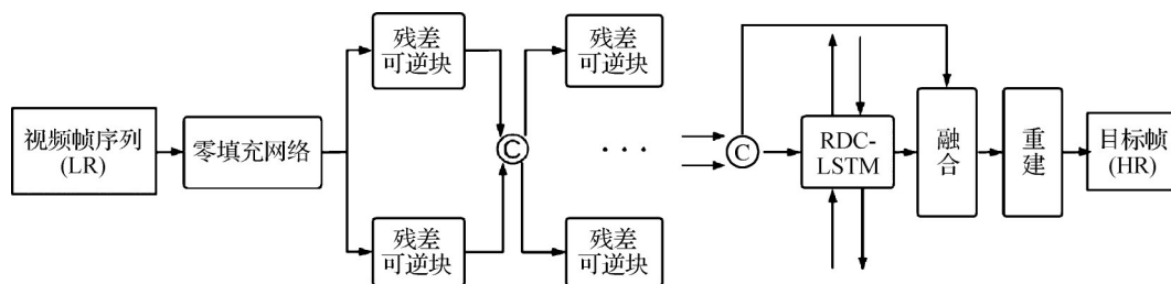
图 30 RISTN 的网络结构 (Zhu 等, 2019a)
