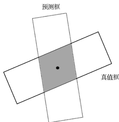
图3 基于交并比进行定位评价的缺点
