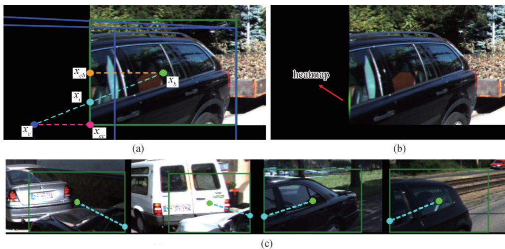
图10 外部物体表示(Zhang等,2021)
