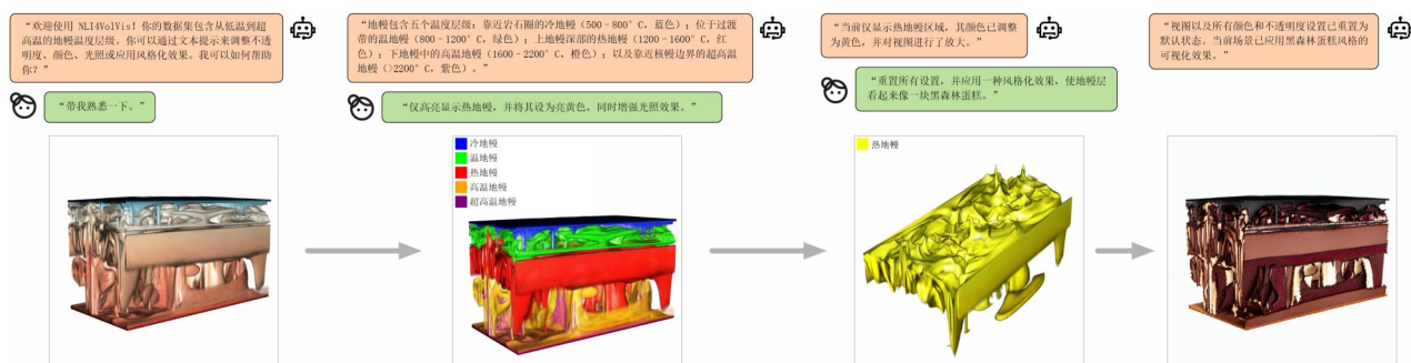
图2 基于自然语言的体数据可视化系统NLI4VolVis在地幔温度场数据集上的交互示例(Ai等, 2025)
