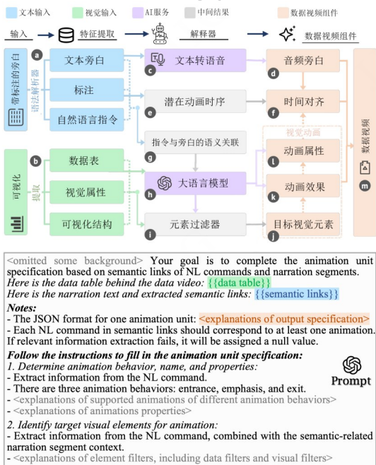
图4 从用户标注中自动合成数据视频 (Shen 等, 2025)
