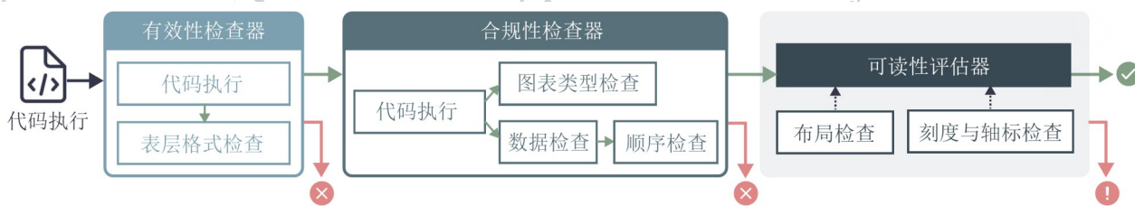
图5 VisEval 评估数据集构建过程主要包含有效性检查器、合法性检查器、可读性评估器等三个主要模块(Chen等,2025)
