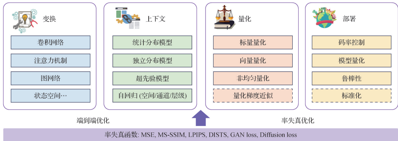
图2 端到端智能图像视频编码核心技术分解
