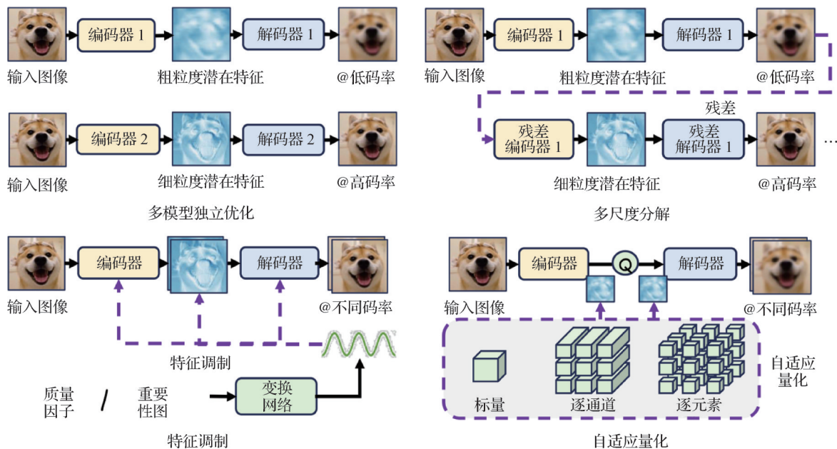
图4 智能图像视频编码可变码率实现方式
