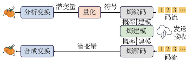
图1 基于VAE的智能编码方案结构图
