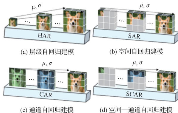
图 3 上下文建模
