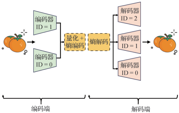
图6 基于多分支设计的 JPEG AI 架构
