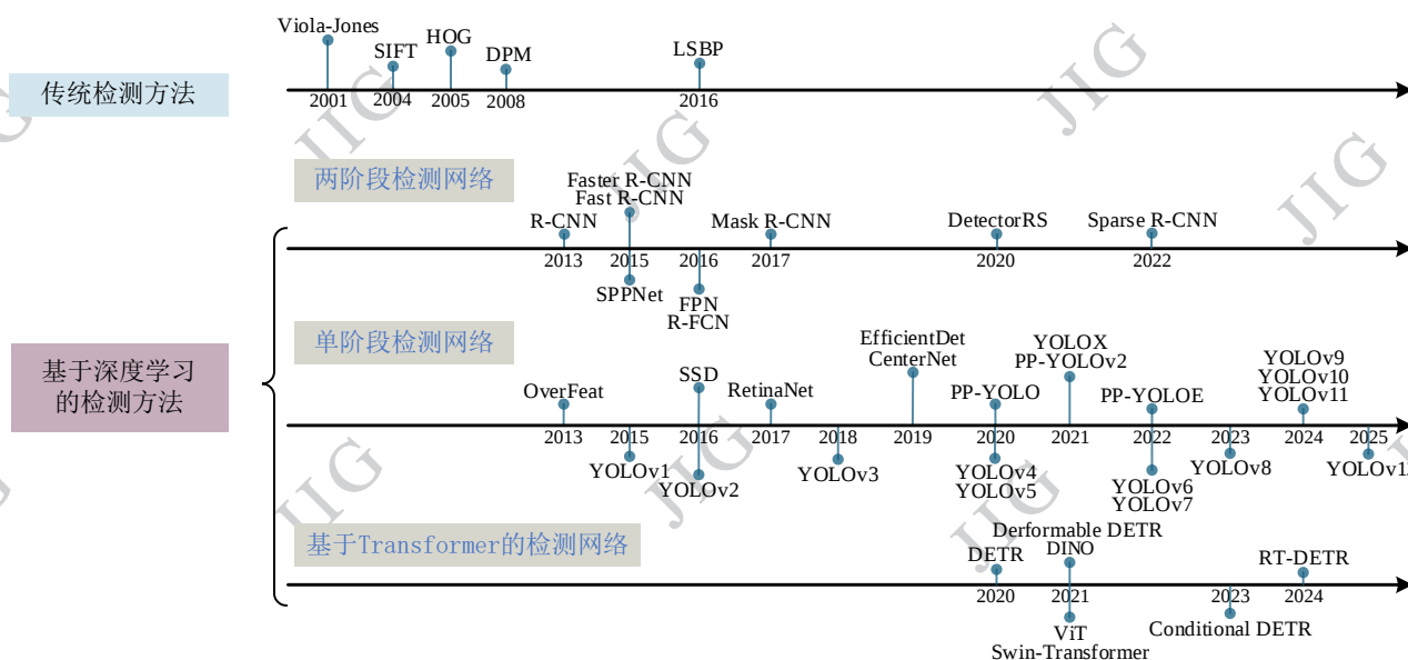
图5 目标检测网络发展脉络图
