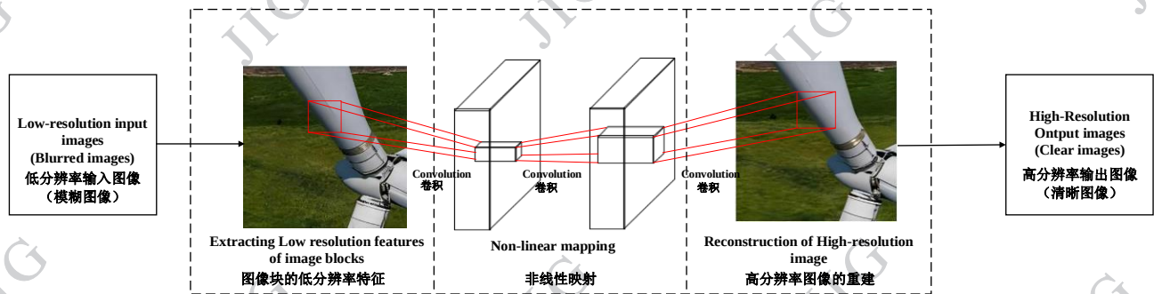
图4 利用SRCNN提高图像质量(Sarkar等,2021)
