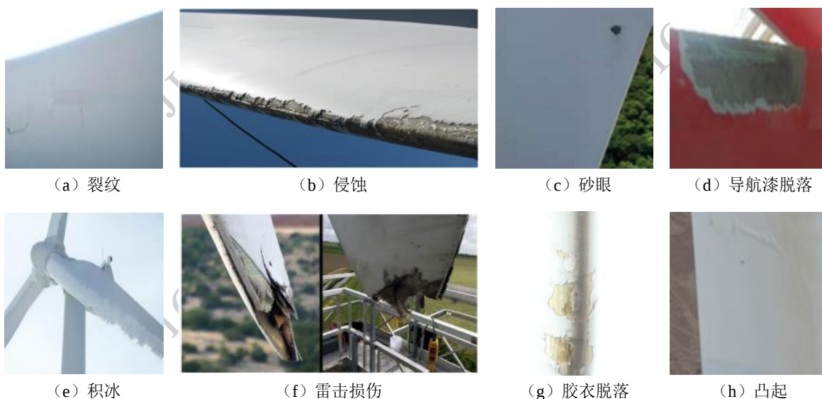
((a) crack;(b) erosion;(c) pinholes;(d) coat peeling;(e) icing;(f) lightning damage;(g) gelcoat peeling;(h) blistering)
