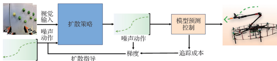
图7 VLA-AN工作流程
