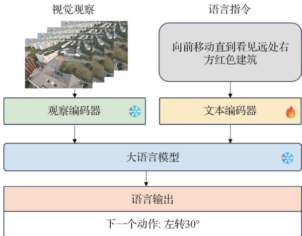
图 4 Navid 结构 Fig. 4 The architecture of Navid
