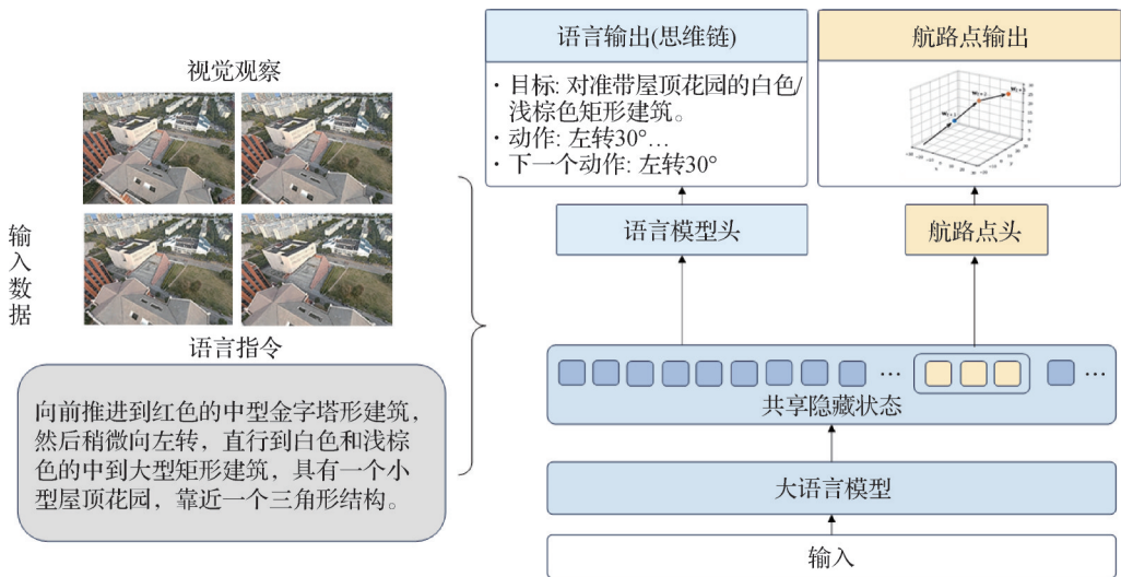
图5 FreeFly-Thinking结构
